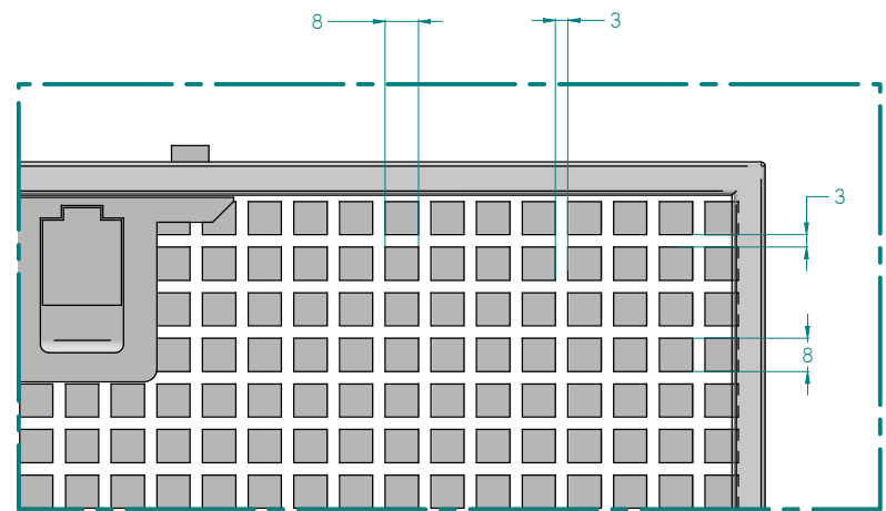
DET. A
