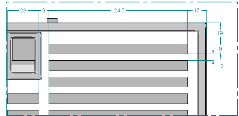
DET. A
